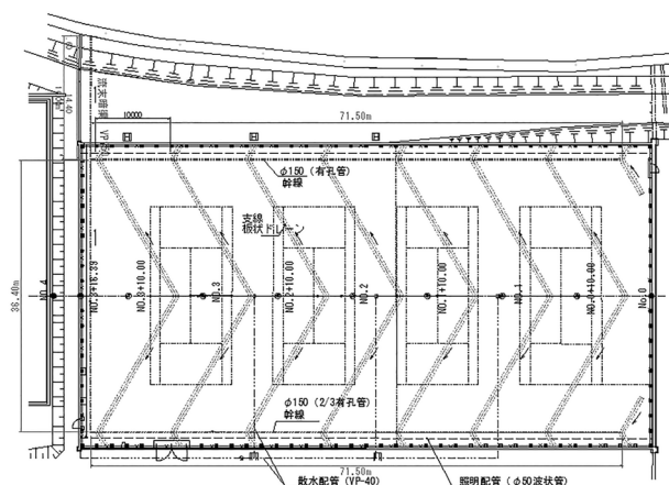
図-2 平面図（排水工）
