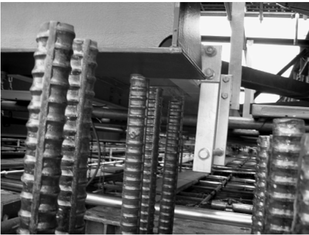
写真-7 反力壁と検査路受台の干渉
