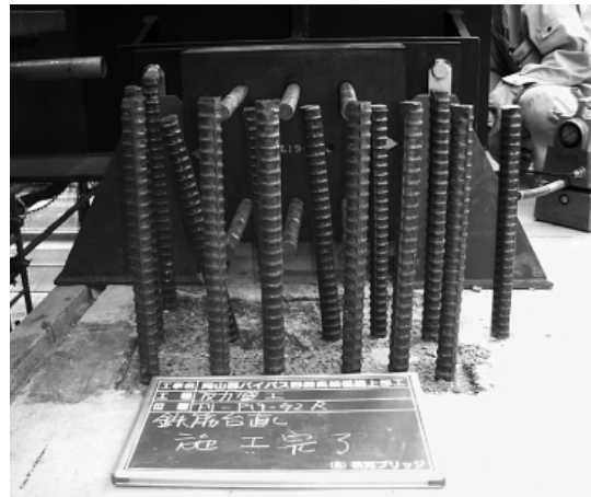
写真-2 鉛直鉄筋の曲げ加工
