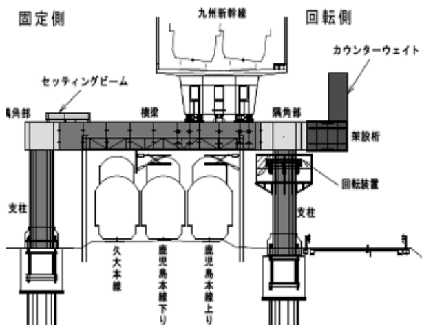
図-3 設備全体図
