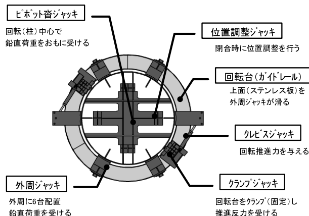
図-4 回転装置の仕組み
