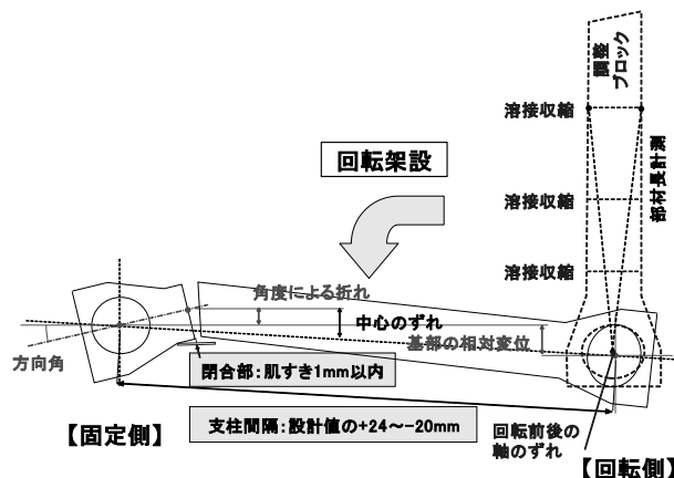
図-5 管理ポイント(平面)
