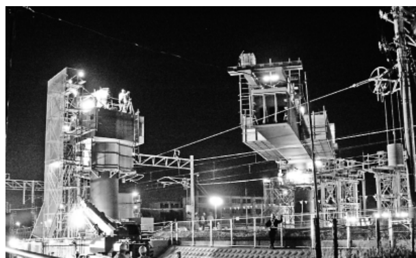
写真-3 回転架設状況
