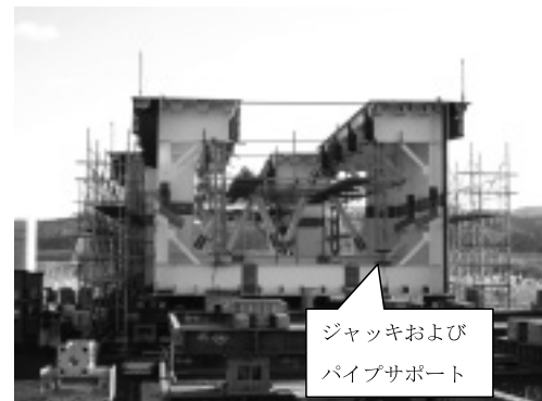
写真-6 桁落とし込み時ジャッキ
