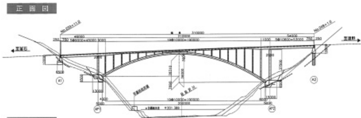
図-2 正面図
