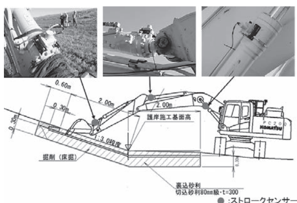
図-2 掘削断面
