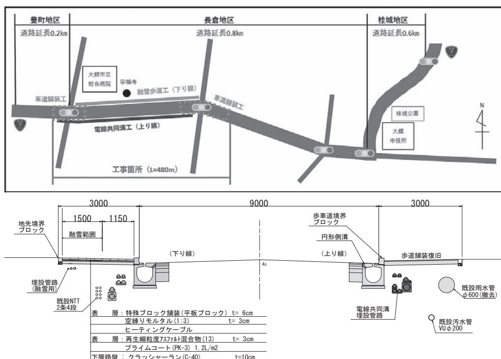
図-1 事業位置図及び標準横断面図
