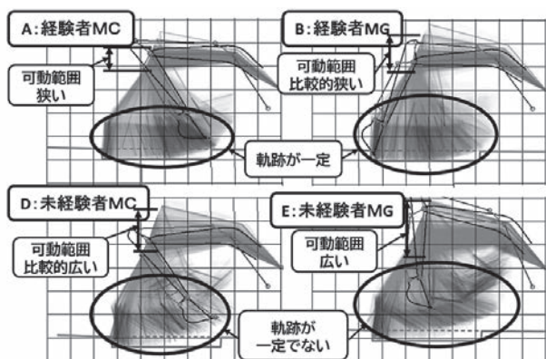
図－4 アーム挙動の比較
