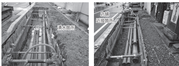
写真－６ 仮設土留めによる土砂崩壊防止
