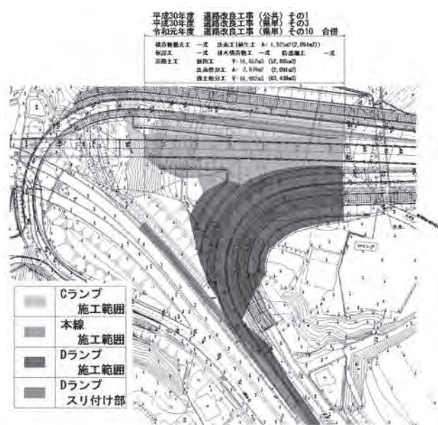
図-1 竣工平面図
