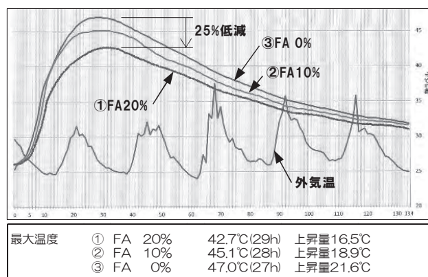
図-4 簡易断熱温度上昇の測定結果
