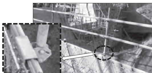
図-8 堤体中間地点：専用金具を用いて転落防止施設設置対策
