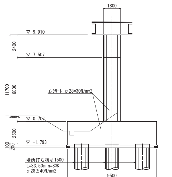
図－3 側面図
