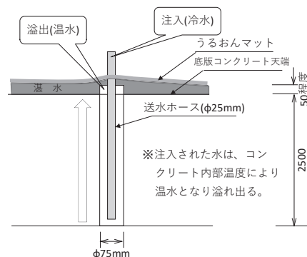
図－9 湛水養生概要
