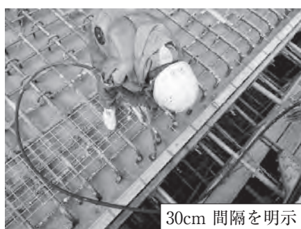
図-11 小径バイブレーターによる締固め
