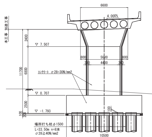
図－2 正面図
