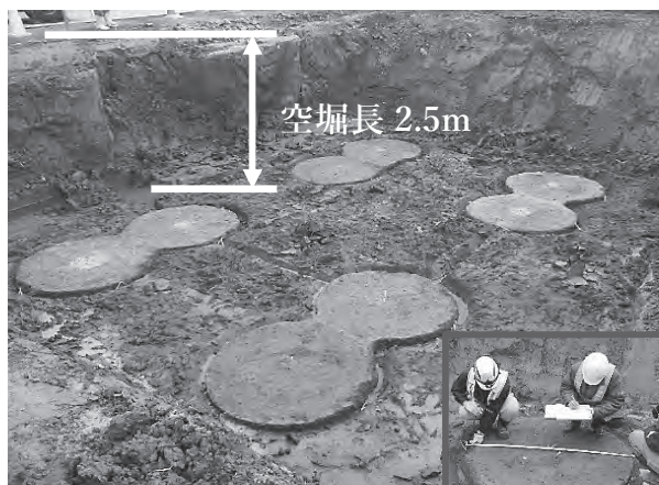
図-2 RMP-MST工法 杭頭出来形確認状況
