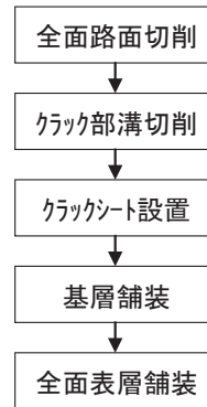
図－６ 施工順序・施工状況写真
