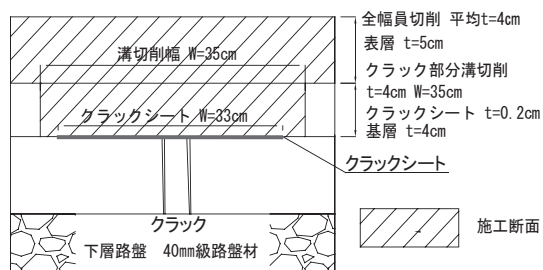
図-4 施工断面図
