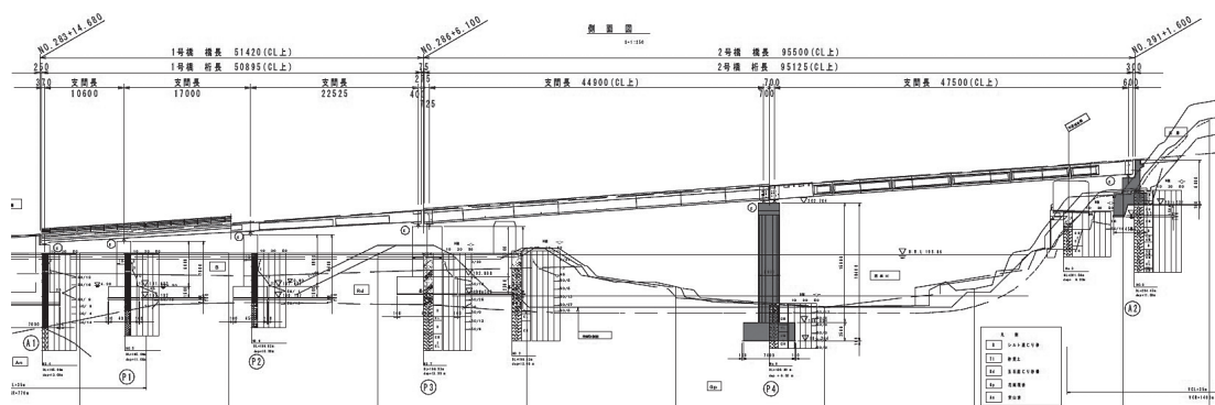
図－1 側面図
