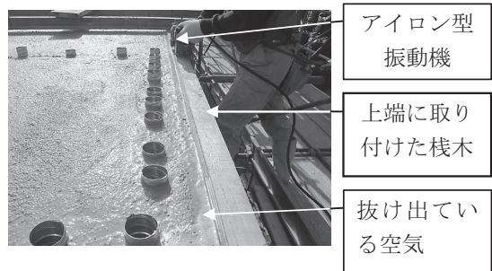
図-5 気泡除去状況
