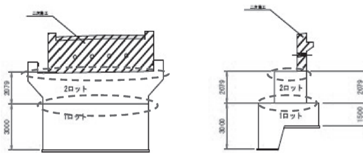
図-2 A2橋台 打設ロット図
