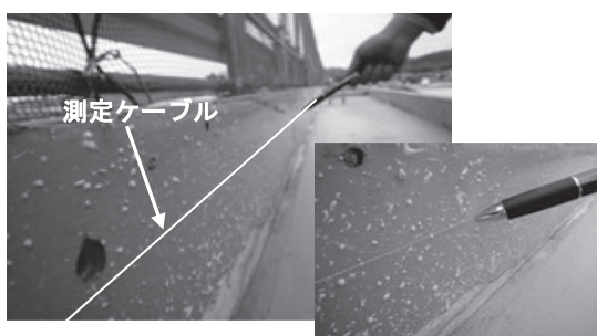
図-6 OFC設置状況
