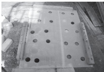
図-4 原寸フィルムによる確認
