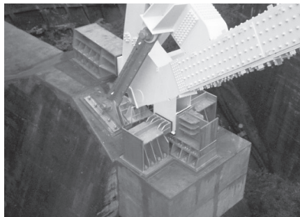
図-6 支柱等基部補強完了
