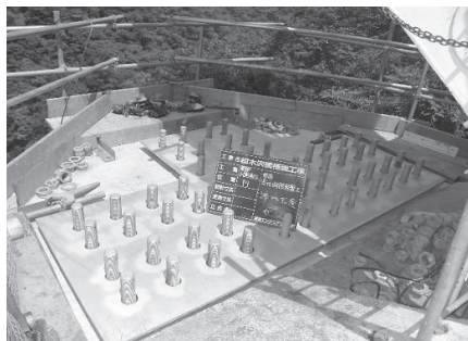
図-5 補強材（プレート）設置完了
