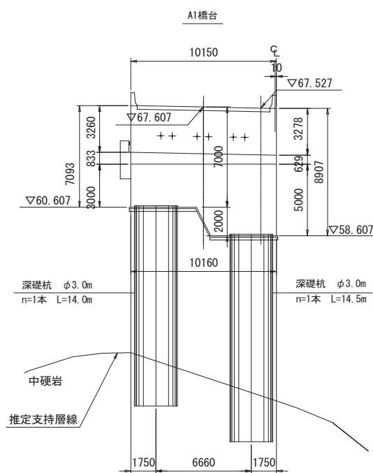
図－2 A1橋台構造図
