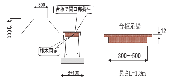
図－２ 足場構造図
