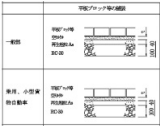
図-2 歩道及び自転車道の舗装構成
