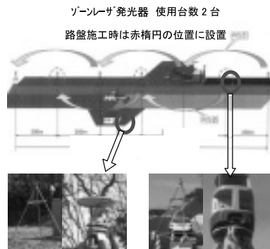
図-4 GPS基地局・発光器設置図
